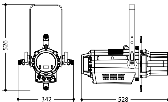
Disegno tecnico
